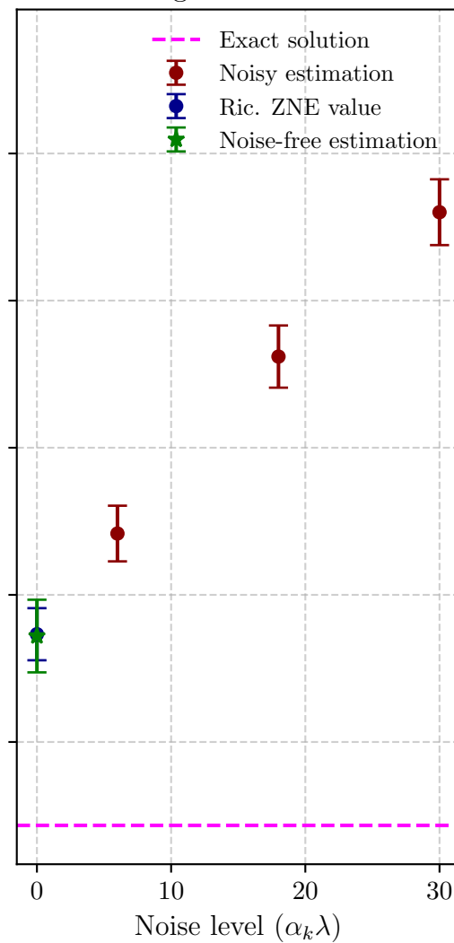
Ising ansatz ric-3
